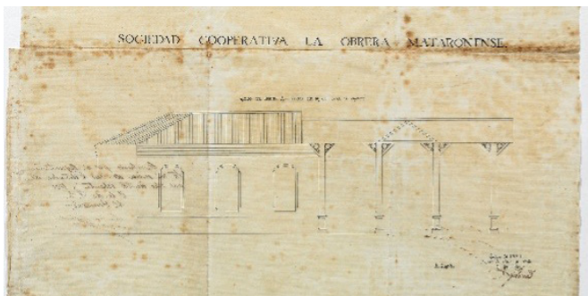
Antoni Gaudí , Barcelona, juliol de 1883. Alcat de la porteria amb habitatge i la porxada . Tinta sobre tela de plànol. Arxiu Comarcal del Maresme. Fons Ajuntament de Mataró ACM70-1-T2-2029
