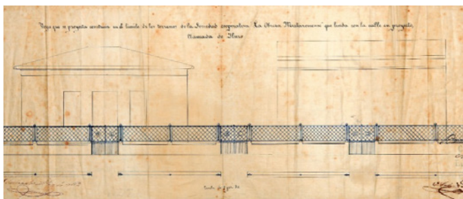
Antoni Gaudí, Barcelona, 26 de juliol de 1878. Alçat de la reixa dels límits del terreny de l'Obrera. Tinta sobre tela de plànol. Arxiu Comarcal del Maresme. Fons Ajuntament de Mataró ACM70-1-T2-2026.
