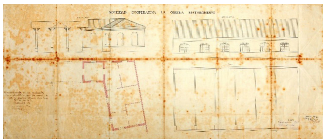
Antoni Gaudí, Barcelona, juliol de 1883. Alçats i plantes dels edificis A i B (la porteria amb habitatge i la nau de blanqueig de cotó). Tinta sobre tela de plànol. Arxiu Comarcal del Maresme. Fons Ajuntament de Mataró ACM70-1-T2-2030.
